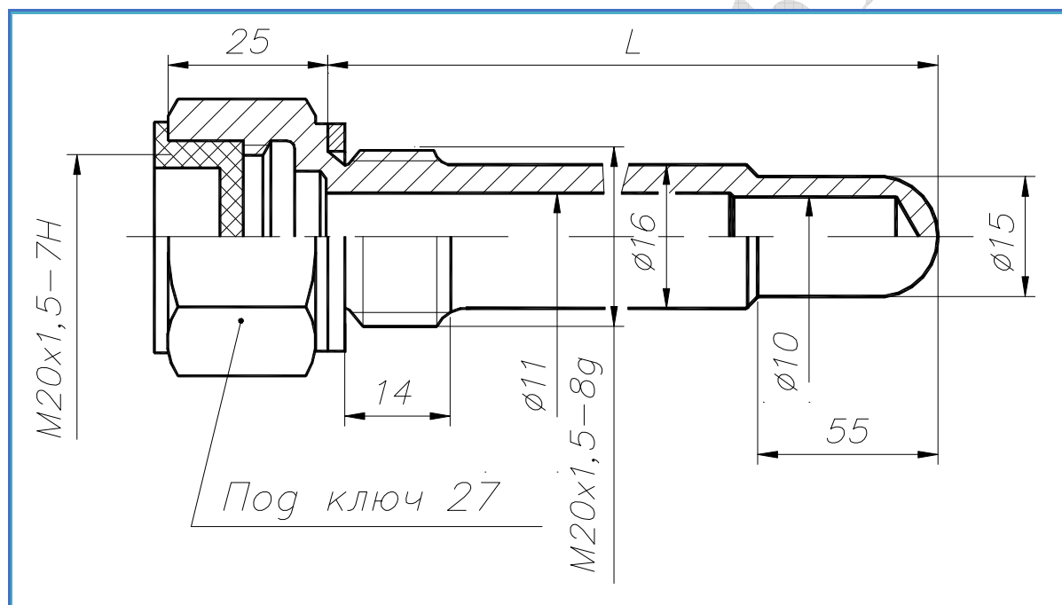
Габаритный чертеж
